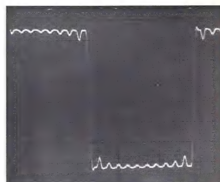
een blokgolf van 1002 Hz uit de DCC-speler
